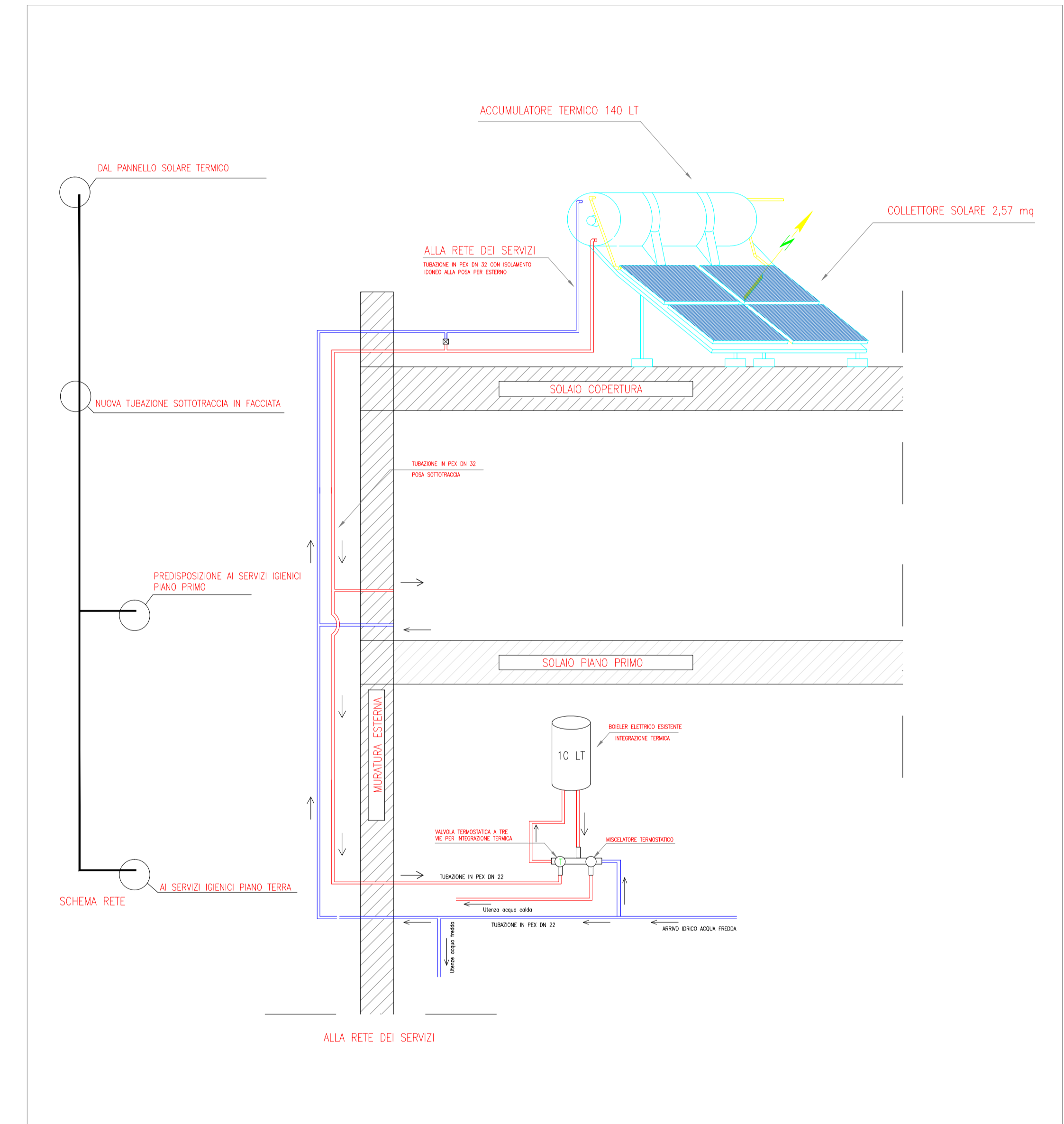
SCHEMA FUNZIONALE DEL SISTEMA SOLARE TERMICO
