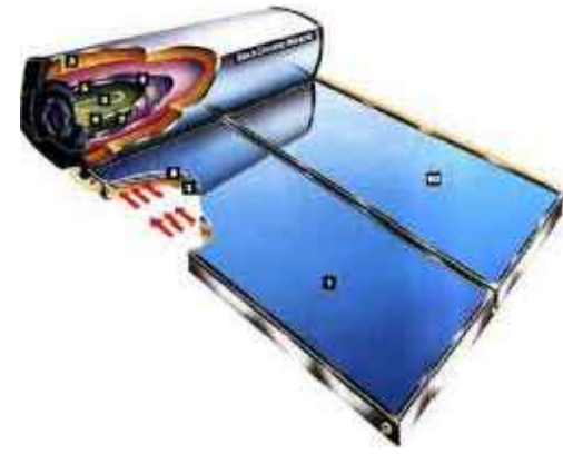
SEZIONE SOLARE TERMICO CIRCOLAZIONE NATURALE
