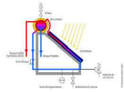
SCHEMA FUNZIONALE
